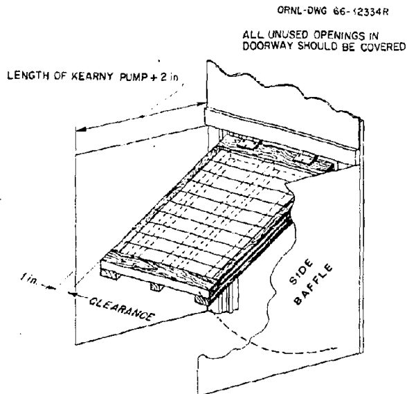
Fig. B-23. Side baffles.
